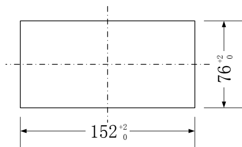
单表开孔尺寸
