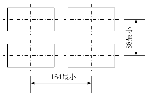
集装表开孔尺寸
